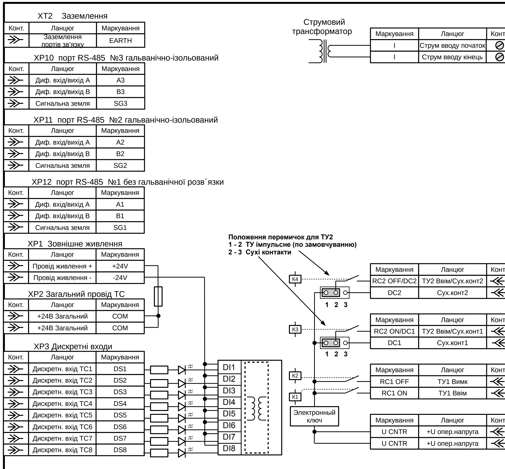
Схема внутрішніх ланцюгів модуля MBV-8-4-I
