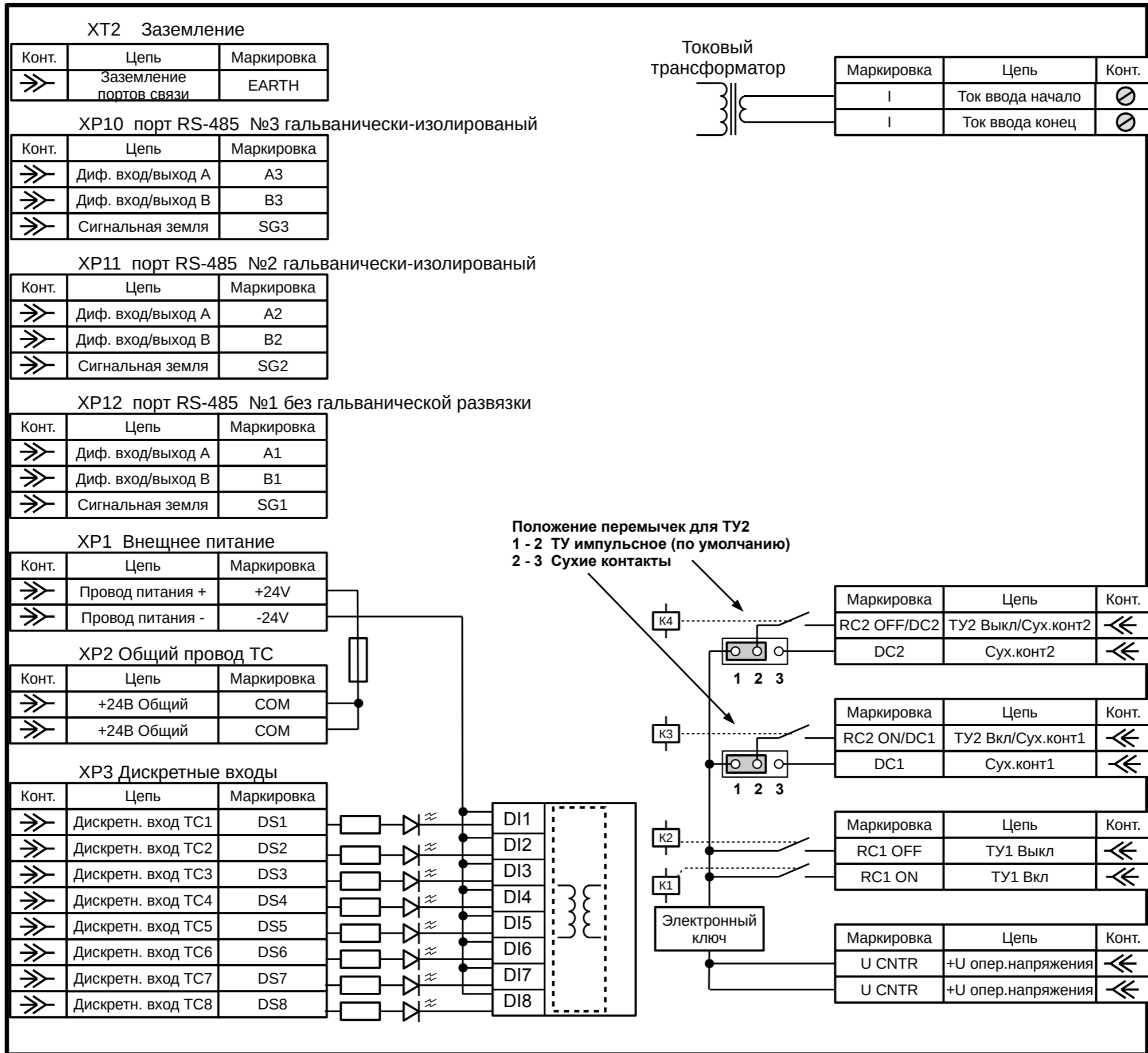
Схема внутренних цепей модуля MBV-8-4-I
